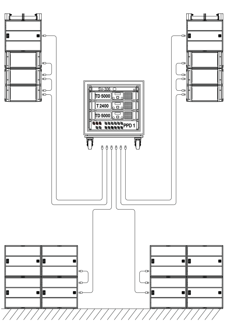
Konfiguration/System D
