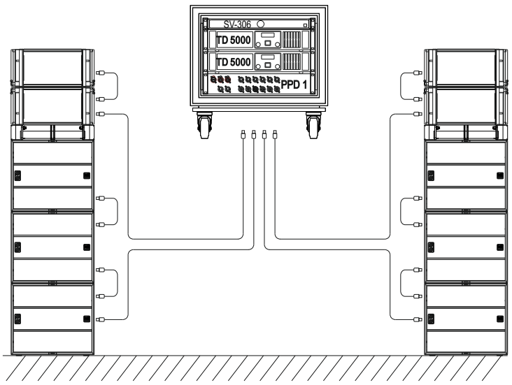
Konfiguration/System B
