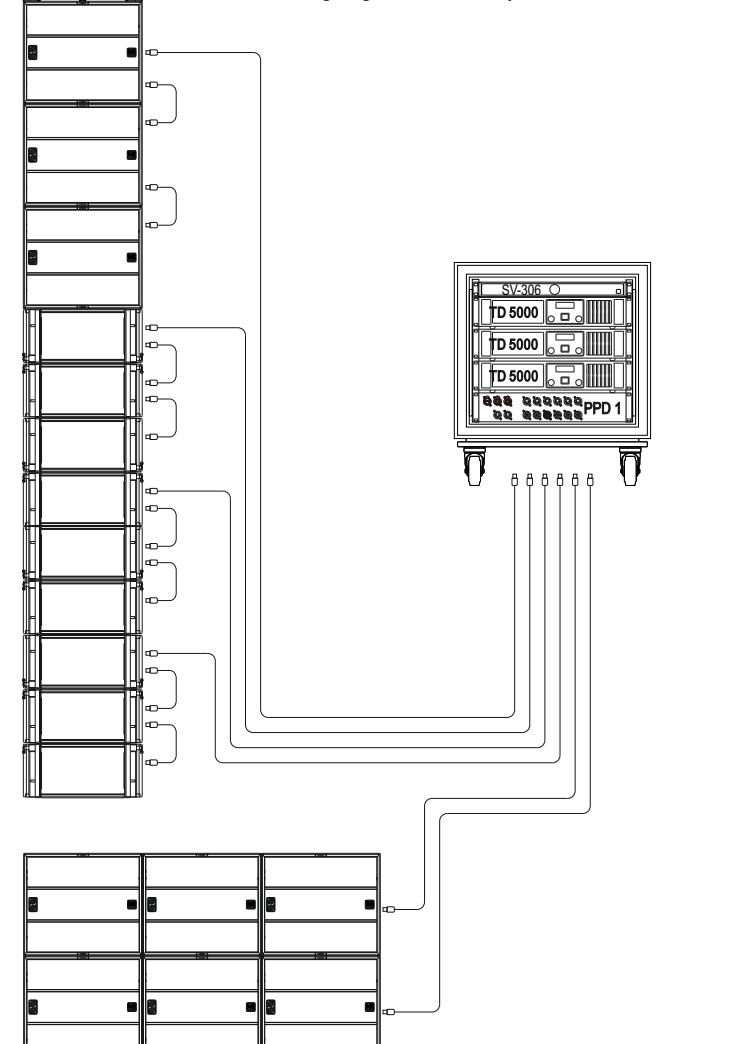
Konfiguration/System G
