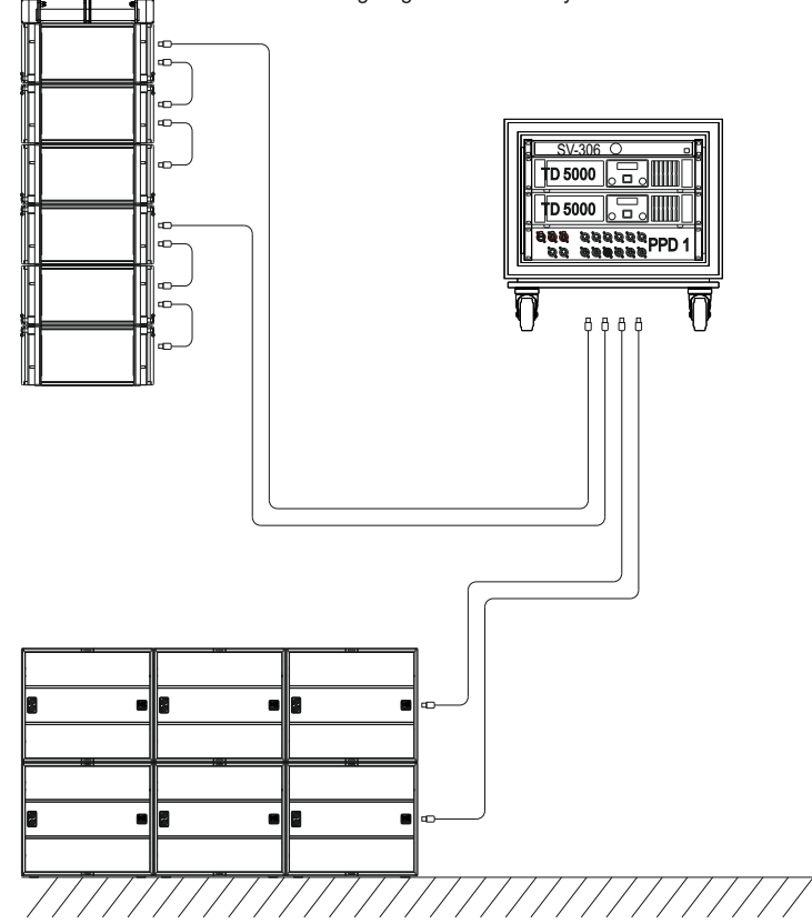
Konfiguration/System F
