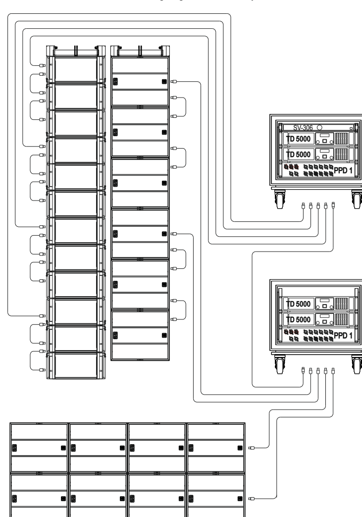
Konfiguration/System H
