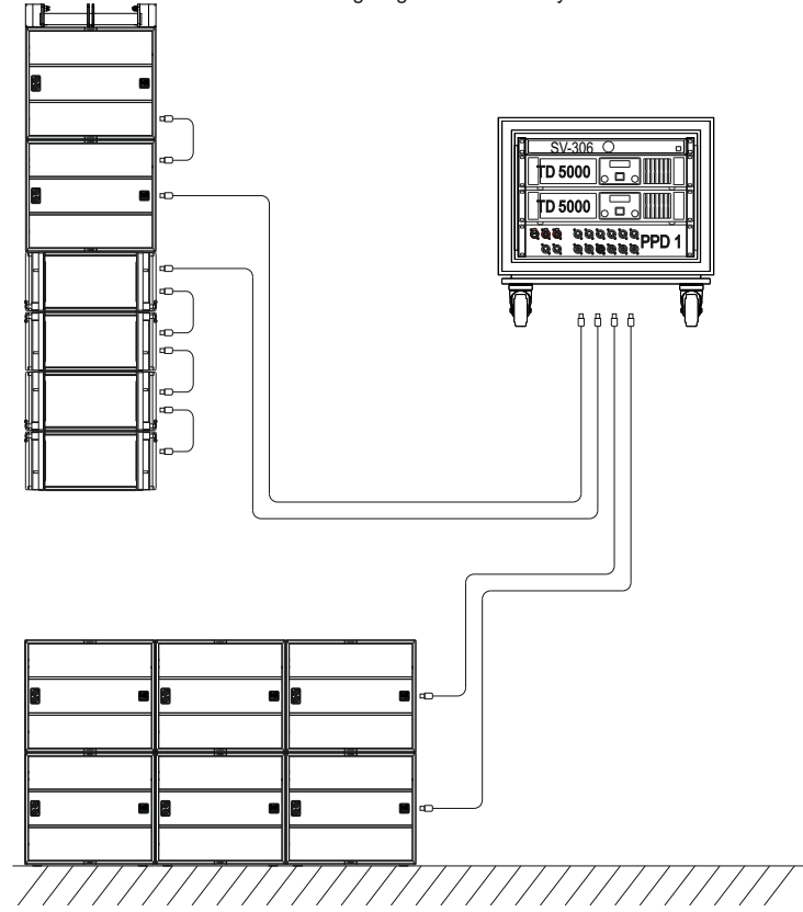
Konfiguration/System E
