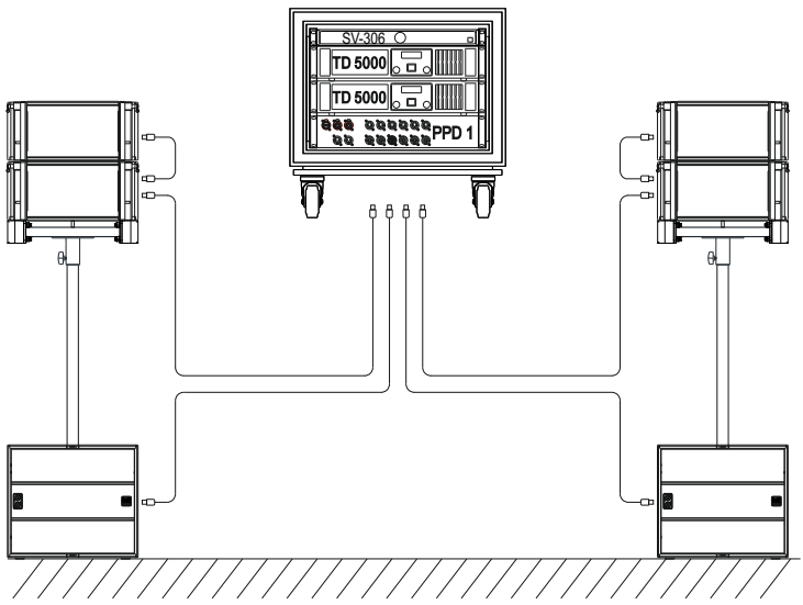
Konfiguration/System A
