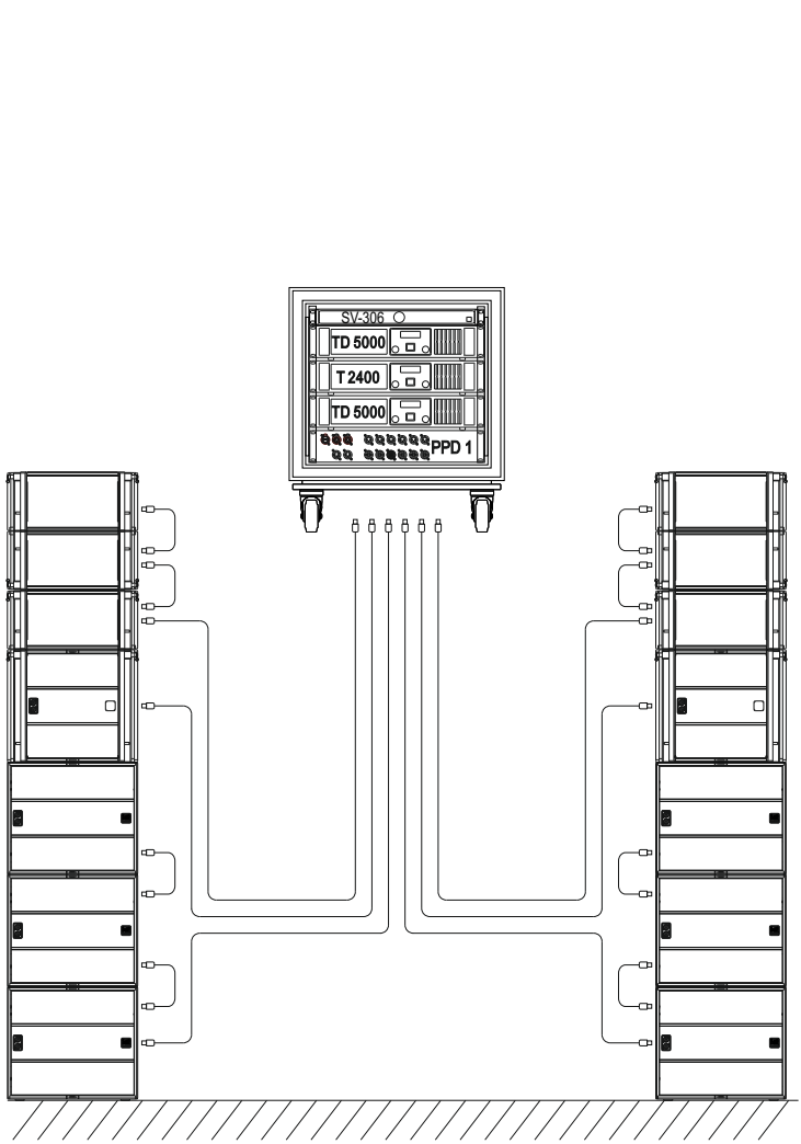
Konfiguration/System C
